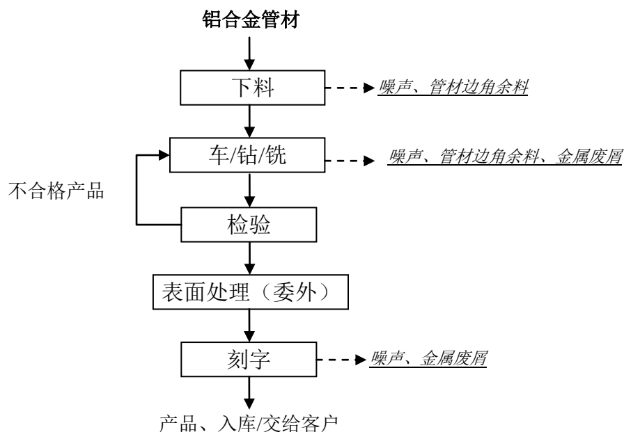
图 5-2 项目生产工艺流程及产污环节
